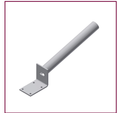
Leuchtausleger Form A Durchmesser 60,3 mm, Länge ca. 500 mm, Rohr 15° schräg angeschweißt, 1 Kabeldurchgangslangloch 16×40 mm, Befestigungswinkel Stärke 8 mm
