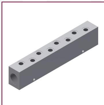
Luftverteiler mit 8 Ausgängen, 1 Eingang Innengewinde G 3/4", 8 Ausgänge Innengewinde G 1/4"
