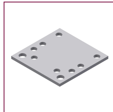
Befestigungsplatte für Leuchtenständer zum Befestigen am Geländer, 120×120×6 mm
