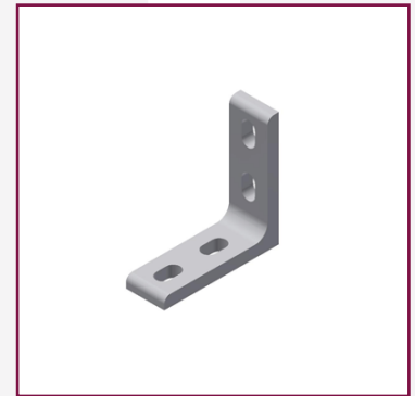
Haltewinkel Nr. 998, Größe 40 Befestigungsteil für U-Stahl 65 mm, Abmessung 120×40×120 mm, Stärke 13 mm, mit 4 Langlöchern 14×25 mm
