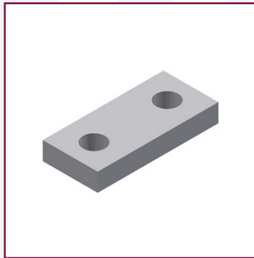
Unterlage für Leuchtenständer Abmessung 30×10×66 mm, zum Befestigen an Rohrgeländern mit Rundstahlbügel, aus Flachstahl
