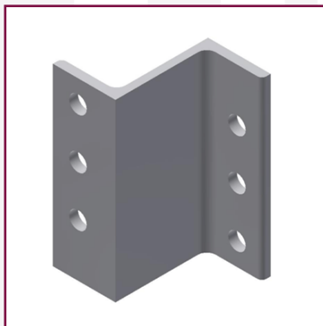
Unteres Zwischenteil EMS-Teil, zum Befestigen an der Treppenwange, aus Z-Stahl 80×140 mm
