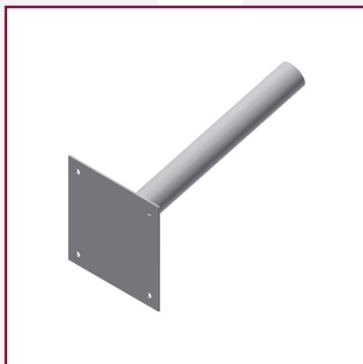
Leuchtausleger Form B Durchmesser 60,3 mm, Länge ca. 500 mm, Rohr 15° schräg angeschweißt, 1 Kabeldurchgangslangloch 16×40 mm, Befestigungsblech Stärke 4 mm mit 4 Bohrungen
