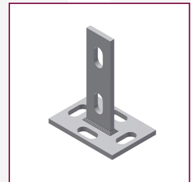
Fußplatte für H-, T- und U-Stiele aus Flachstahl 100×30×5 mm und 80×5 mm
