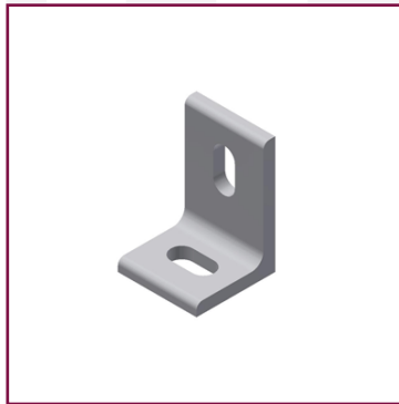
Haltewinkel Nr. 905, Größe 4 Befestigungsteil für U-Stahl 40×20 mm, Abmessung 60×40×40 mm, Stärke 6 mm, mit 2 Langlöchern 11×22 mm
