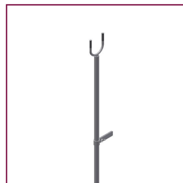
Stützgabel für umklappbaren Leuchtenständer DN65
