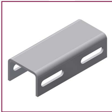
Abstandshalter für Leuchtenständer am Geländer DN32, in U-Form 140×60×40 mm
