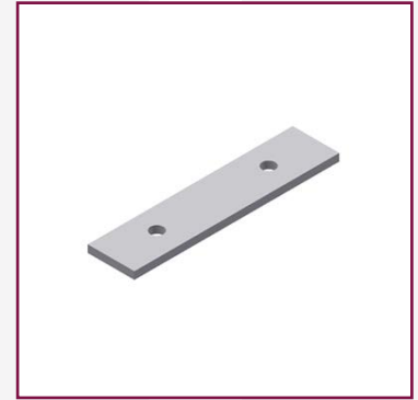
Abstandshalter 952 Befestigungsteil für Rohre Ø 12 mm, Länge 110 mm, aus Bandstahl 25×4 mm
