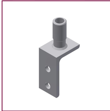
Tragkonsole für Leuchtenständer DN32
