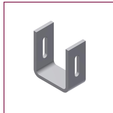
Befestigungsteil für Luftverteiler gekantetes U mit 55 mm Schenkellänge, Materialbreite 25 mm, Stärke 4 mm, mit 2 Langlöchern 6,5×26 mm
