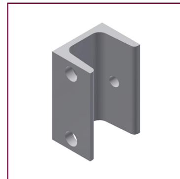
Befestigungsteil zur Befestigung der Leuchte am Gewinderohr, aus U-Stahl 50×76 mm
