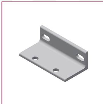
Haltewinkel Nr. 902 Befestigungsteil z.B. für Messumformer, Abmessung 120×60×40 mm, Stärke 6 mm, mit 2 Langlöchern 11×22 mm und 2 Rundlöchern Ø 12 mm
