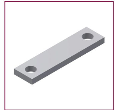
Befestigungsplatte für Leuchtenständer aus Flachstahl, 120×30×8 mm, Lochabstand 94 mm
