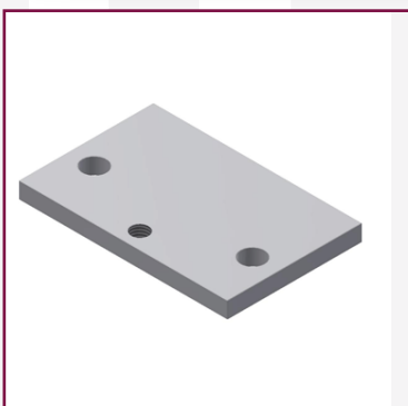
Flachstahlkralle Größe 7 Abmessung 124×80×10 mm mit 2 Löchern Ø 14 mm und Lochabstand 104 mm, 1 Gewinde M12
