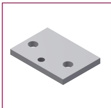
Flachstahlkralle Größe 6 Abmessung 106×80×10 mm mit 2 Löchern Ø 14 mm und Lochabstand 76 mm, 1 Gewinde M12
