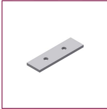
Abstandshalter 951 Befestigungsteil für Rohre Ø 12 mm, Länge 85 mm, aus Bandstahl 25×4 mm
