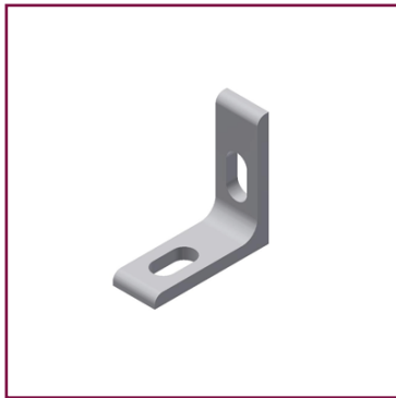
Haltewinkel Nr. 002, Größe 2 Befestigungsteil für U-Stahl 40×20 mm, Abmessung 60×22×60 mm, Stärke 6 mm, mit 2 Langlöchern 11×22 mm
